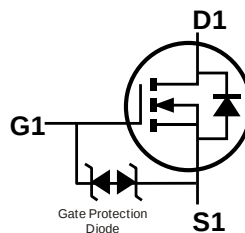
Q1 N-CHANNEL
